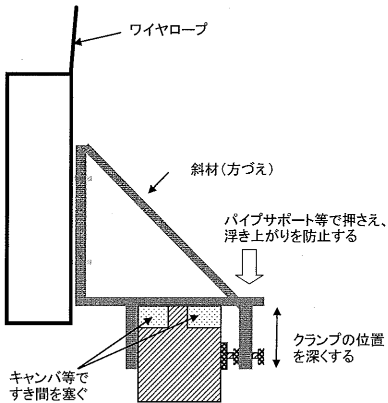
図2 補強例
