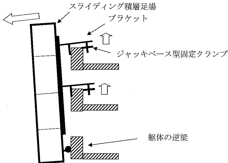
図 落下した足場の推定図
